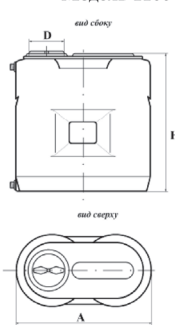
Модель 1100
