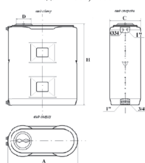
Модели 1500, 2000
