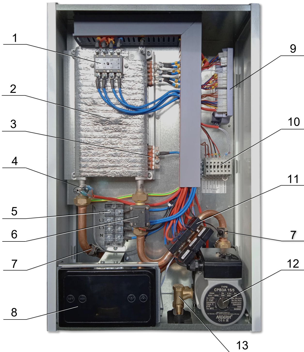
Рис. 1 Общий вид
