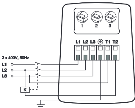
Рис.6. Схема подключения трехфазного насоса
