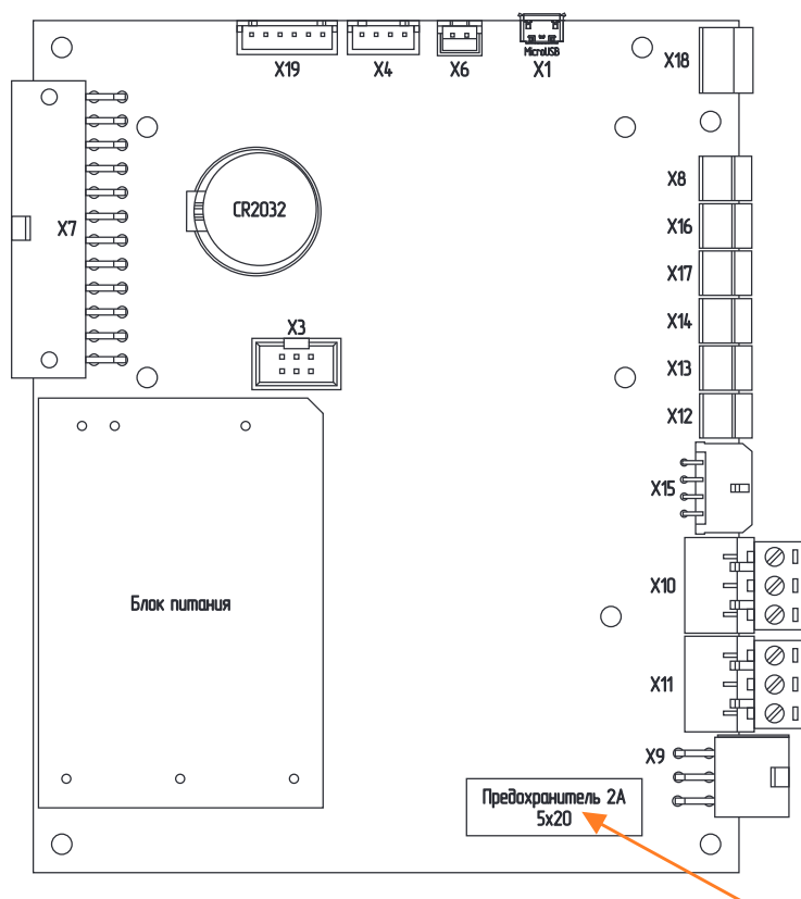
Рис.16 Плата контроллера
